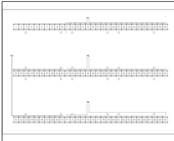
ภาพที่ 2 แสดงตำแหน่งการวางและวงจรย่อยแผงโซลาร์เซลล์บนดาดฟ้าอาคารหอสมุดฯ
