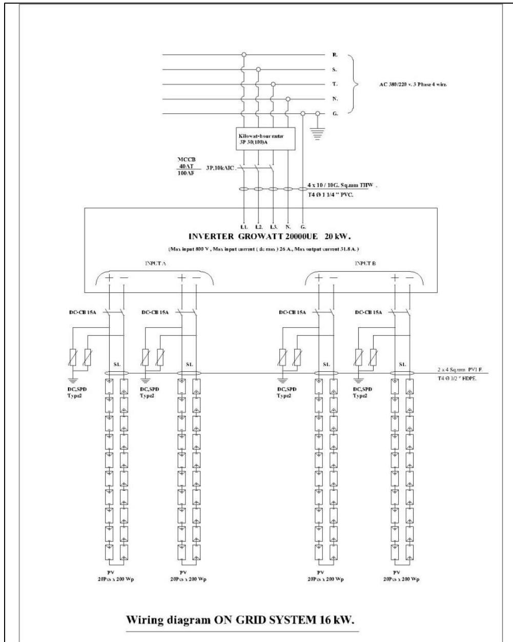
ภาพที่ 1 แสดงภาพ Wiring Diagram ระบบไฟฟ้าโซลาร์เซลล์ติดตั้งฟาร์มอาคารหอสมุดฯ
